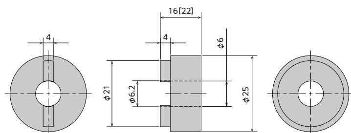
FFD-25SS-**** ([ ]内の数値はFFD-25SW-****の寸法です)
