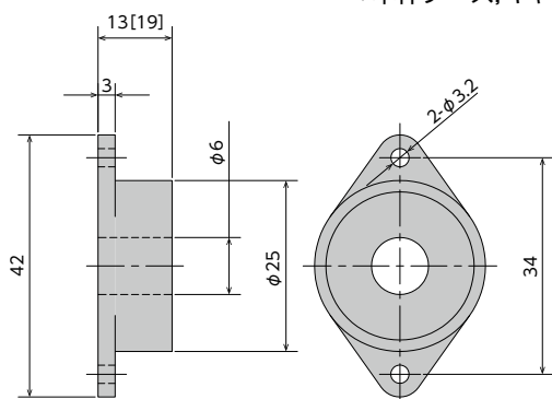
FFD-25FS-**** ([ ]内の数値はFFD-25FW-****の寸法です)
