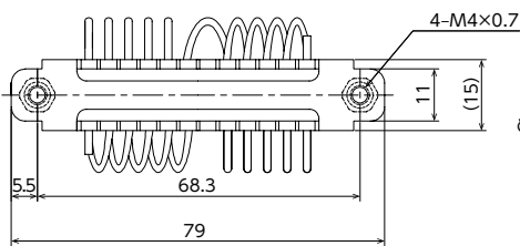
A type(取付部ネジ)
