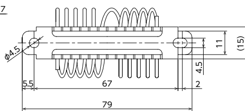
D type(取付部キリ穴)
