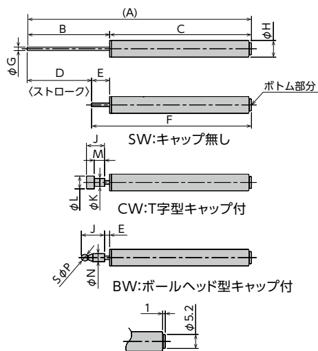
図1 FPD-0725シリーズのボトム形状
