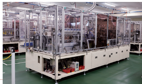
自動組立機
